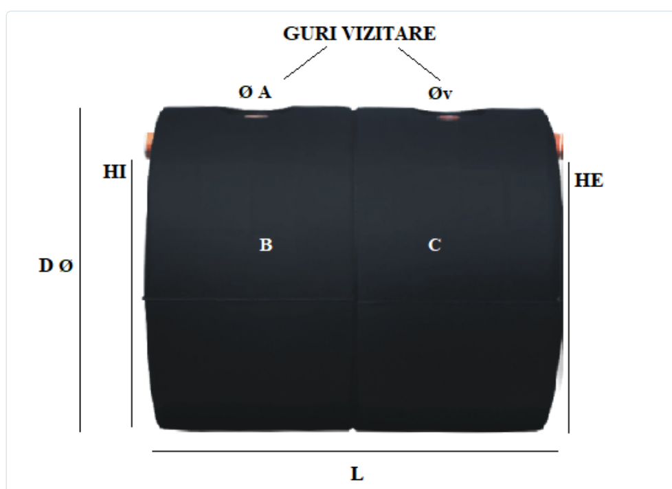
Schemă constructivă — fosă septică bicamerală (secțiune)
